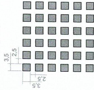
IM pattern No.5 (39%)
