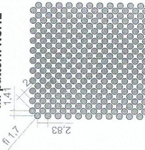
IM pattern No.12
