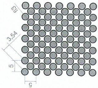
IM pattern No.1 (55%)
