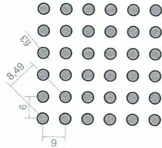
IM pattern No.2 (23%)
