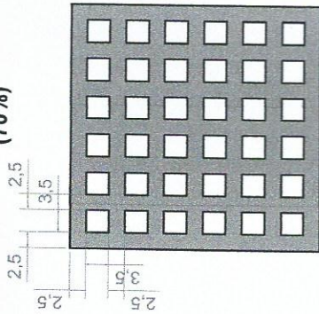
IM pattern No.4 (70%)
