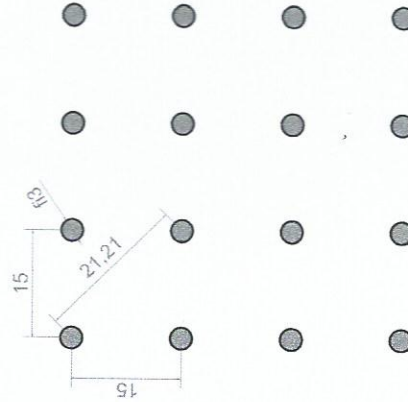
IM pattern No.7 (5%)
