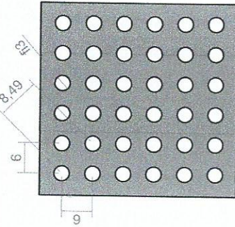
IM pattern No.3 (77%)
