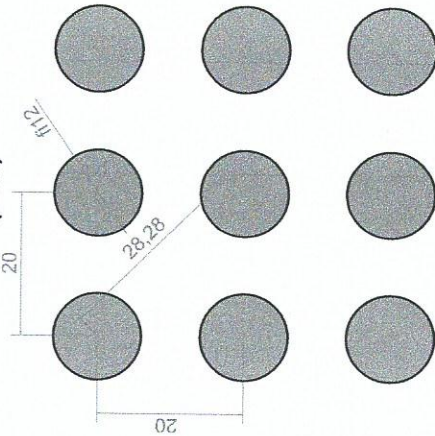
IM pattern No.6 (37%)
