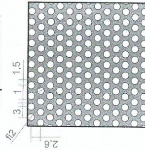
IM pattern No.11
