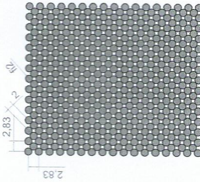
IM pattern No.8 (76%)
